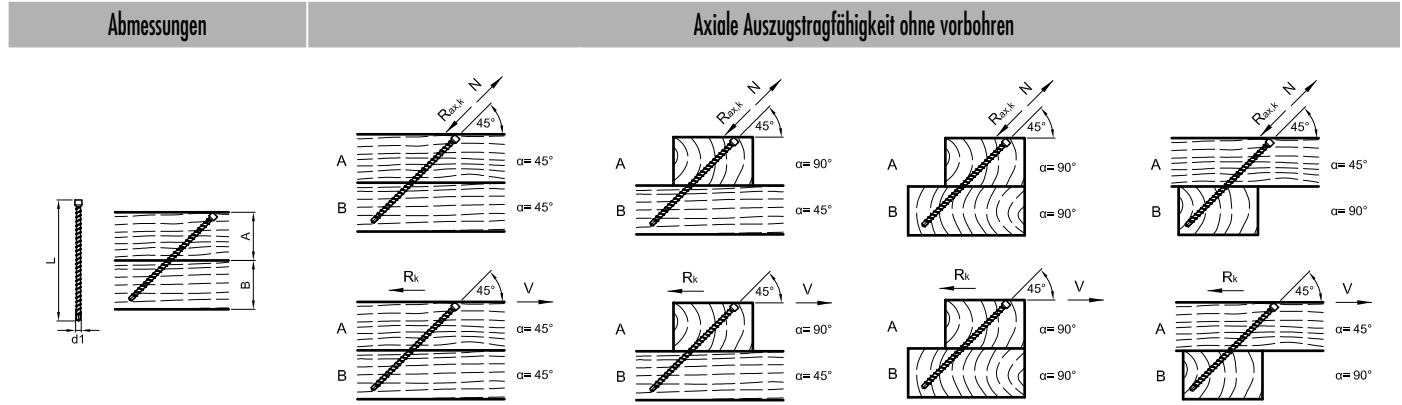
Charakteristischer Wert der Tragfähigkeit der Verbindung R_k nach ETA-11/0024
