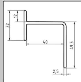
Zeichnung oberes Profil
