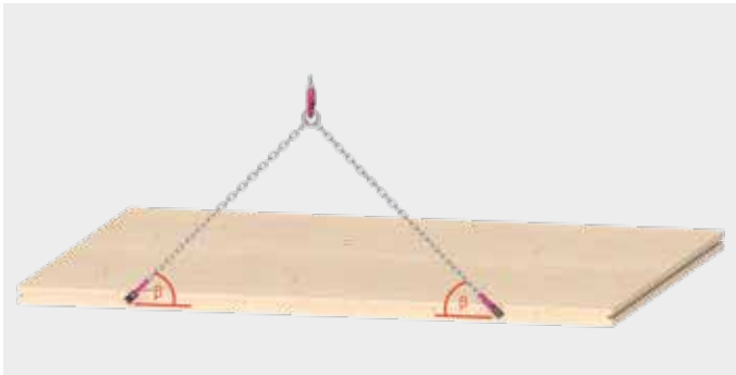
CLT-Wand oder-Träger liegend
