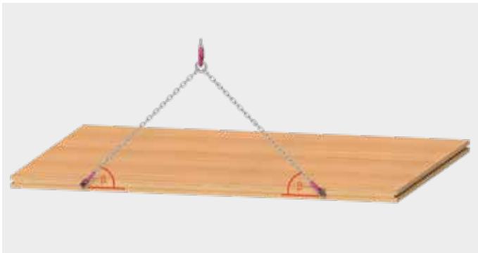
BSH-Wand oder-Träger liegend, Faserverlauf: vertikal
