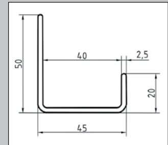
Zeichnung unteres Profil
