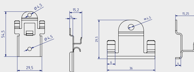
Fassadenclip-Rhombus
