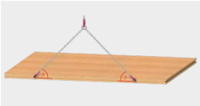
BSH-Wand oder-Träger liegend, Faserverlauf: horizontal
