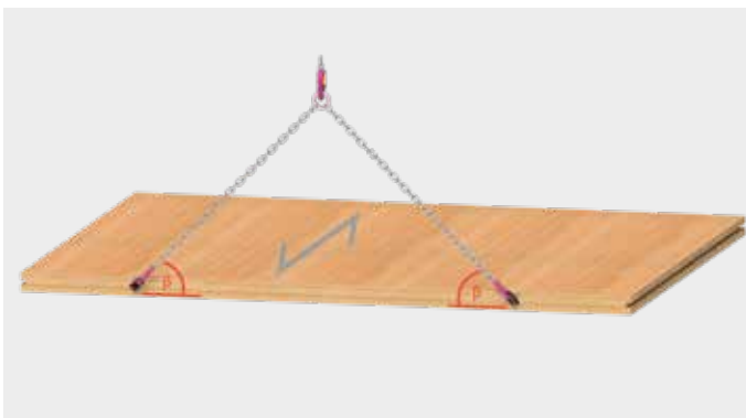
BSH-Wand oder-Träger liegend, Faserverlauf: vertikal
