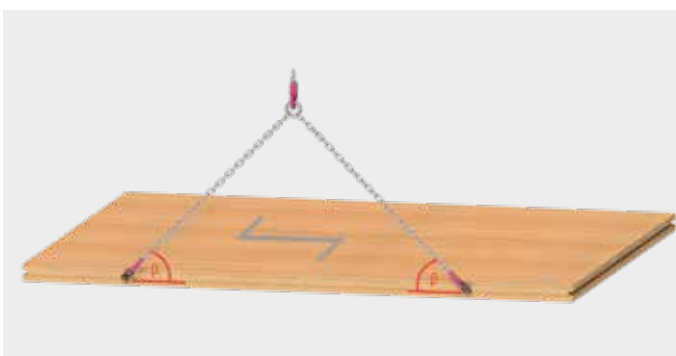
BSH-Wand oder-Träger liegend, Faserverlauf: horizontal
