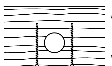
Querzugverstärkung an Durchbruch
