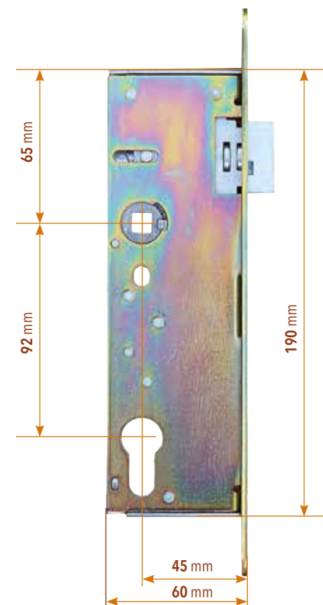
Einsteckschloss für Zauntore mit Ausfräsung
