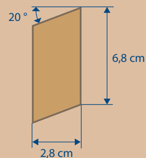
Rhombuszaun Malmö: aus Rhombusprofil Lärche/Douglasie, 2,8 x 6,8 x 180cm, glatt gehobelt, roh, Riegel: 2,5 x 6,5cm
